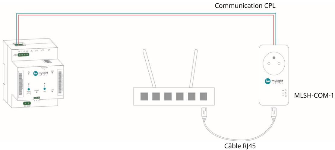
Figure 3 : Schéma de connexion internet via la prise CPL
