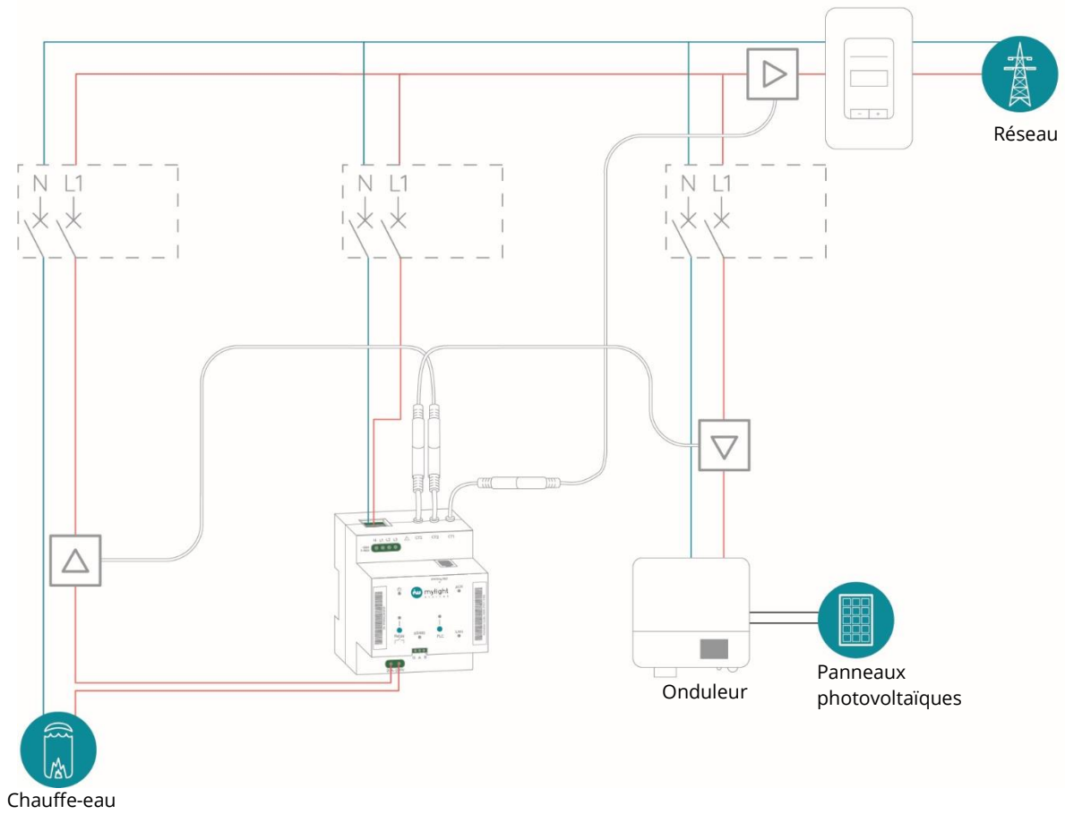
Figure 13 : Exemple d'alimentation monophasée et mesure de production par transformateur de courant
