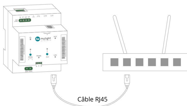
Figure 2 : Schéma de connexion filaire entre MG3 et Box internet
