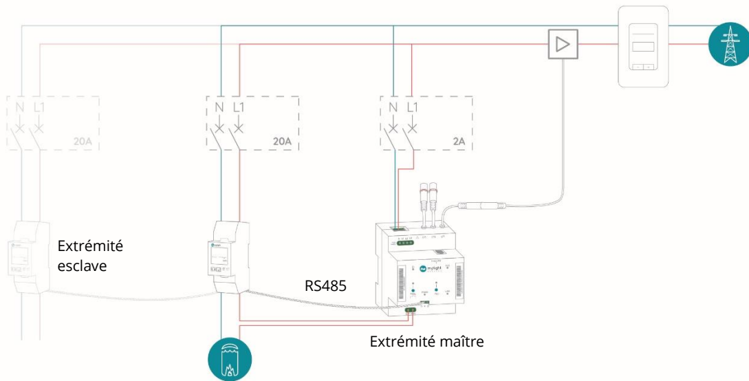
Figure 12 : Exemple de branchement d'appareils RS485
