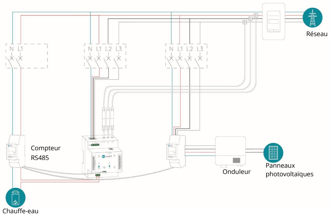
Figure 14 : Exemple d'alimentation triphasée et mesure de production par compteur RS485
