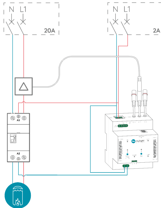
Figure 10 : Exemple de branchement : pilotage d'une charge >20A
