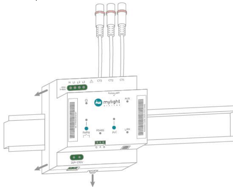
Figure 1 : Instructions de montage mécanique
