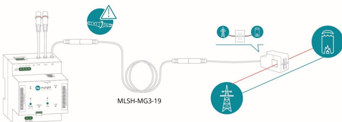
Figure 11 : Exemple d'utilisation de la rallonge et du transformateur de courant
