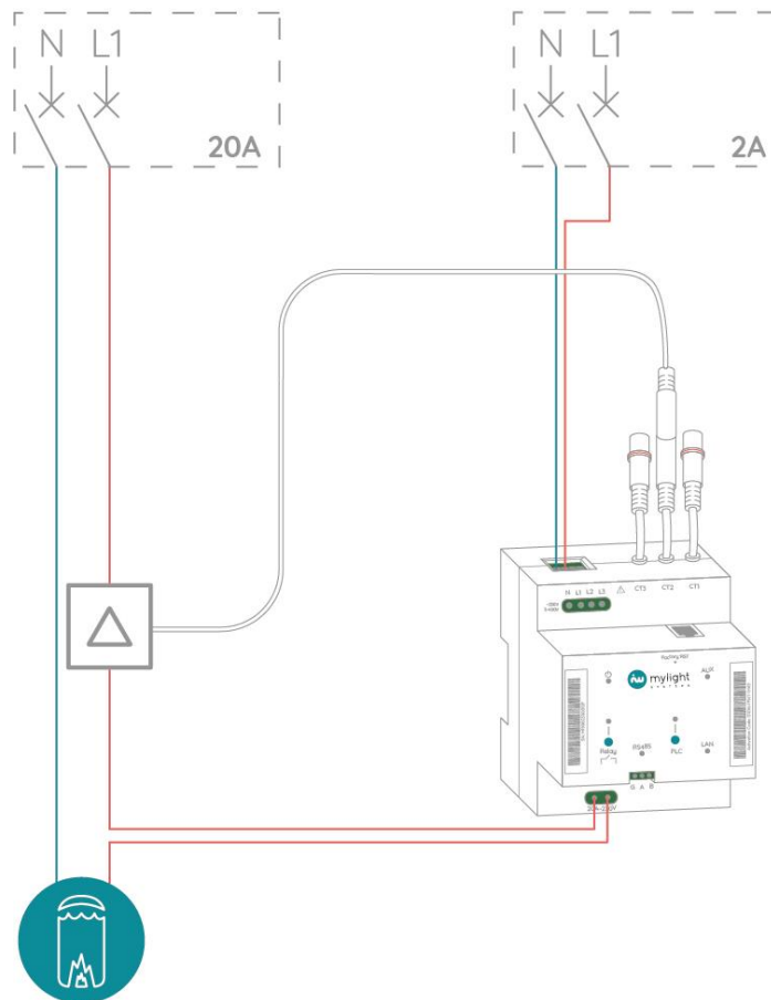
Figure 9 : Exemple d'utilisation pour le câblage du relais
