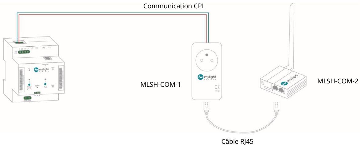
Figure 6 : Connexion internet via le modem cellulaire et prise CPL
